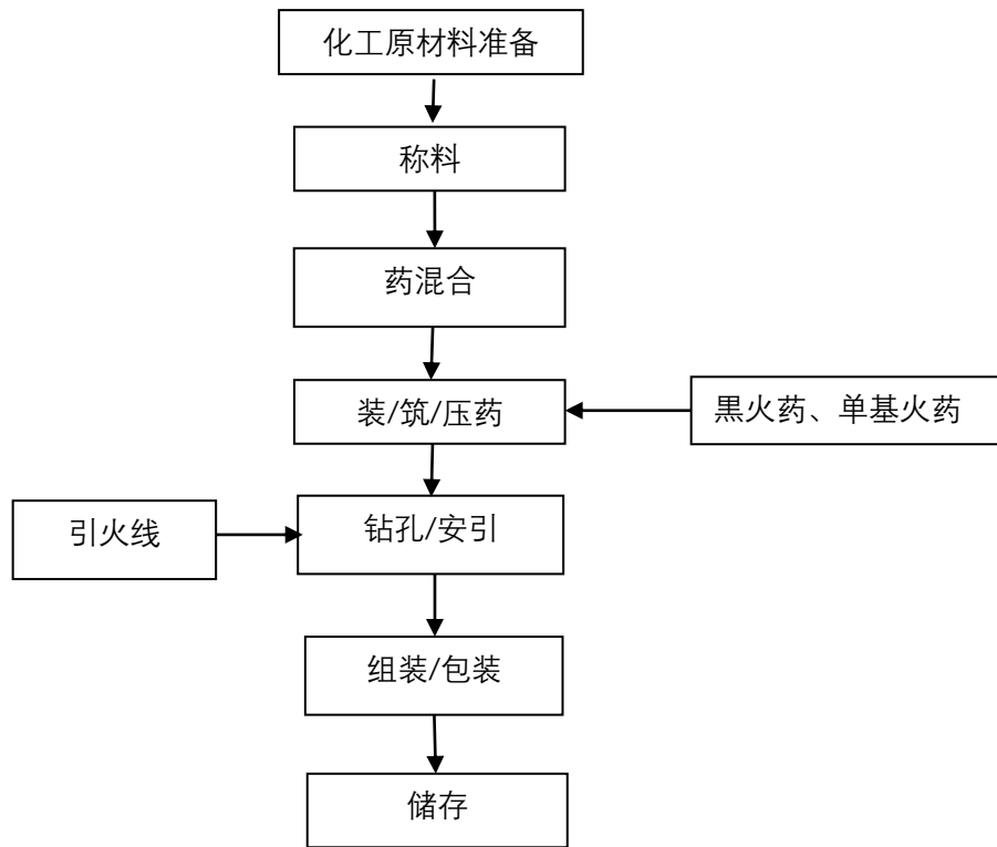
图 2.4-1 喷花类产品生产工艺流程图
